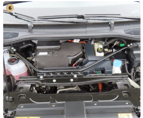
6 Motor A hűtőfolyadék szintje megfelelő.
